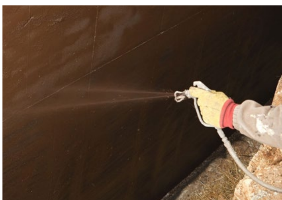
Pose d'un hydrofuge sur des blocs béton
