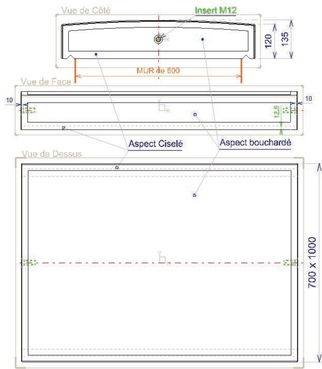
100 x 70 x 12 / 13.5 cm ; 205 kg.
