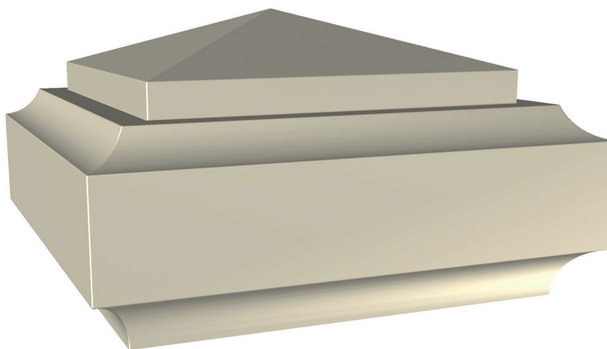
Couronnement diamant Déco pour pilier de : · 40 : 54 x 54 x 27 cm ; 125 kg. · 50 : 61 x 61 x 30.5 cm ; 182 kg.
