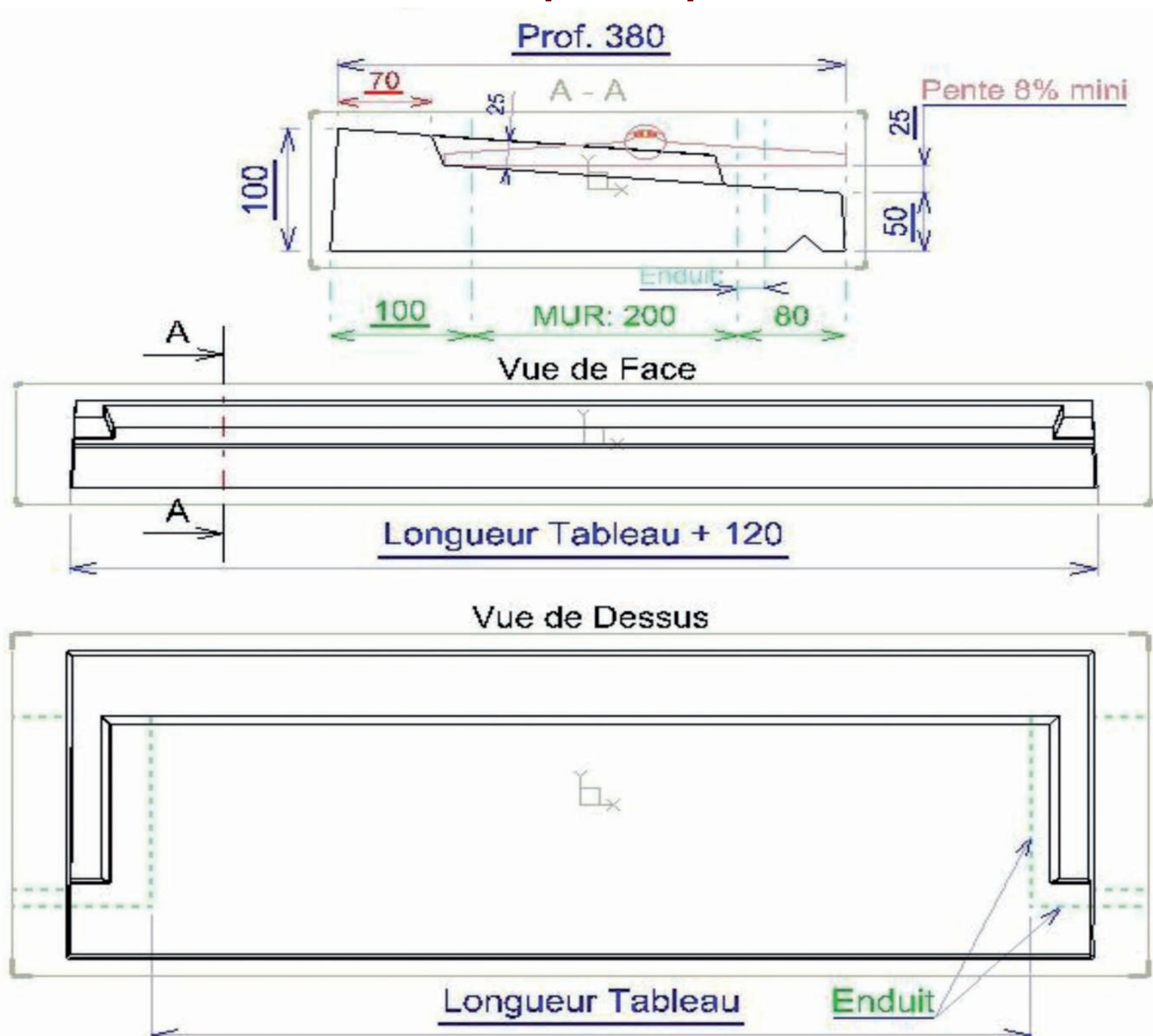
SEUIL de 380 pour : porte-fenêtre
